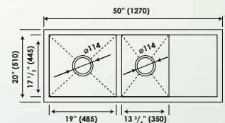
Strainer & Pipe
